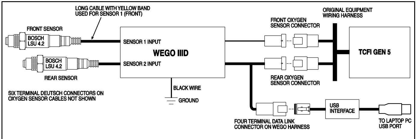
Figure 26 - WEGO Hookup
