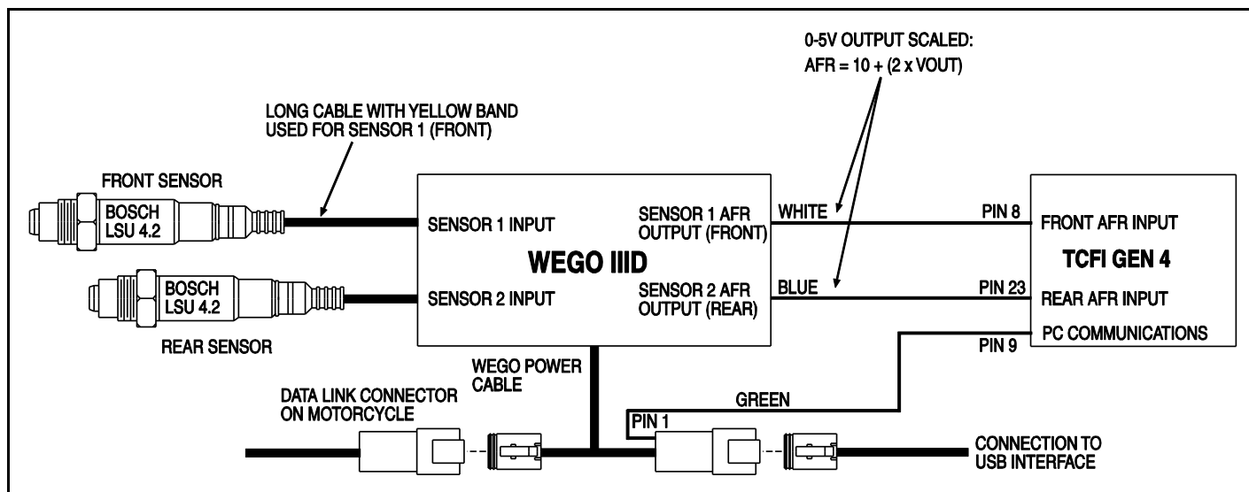
Figure 27 - WEGO Hookup
